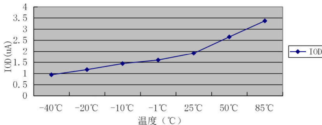
过放自恢复功耗与温度曲线
