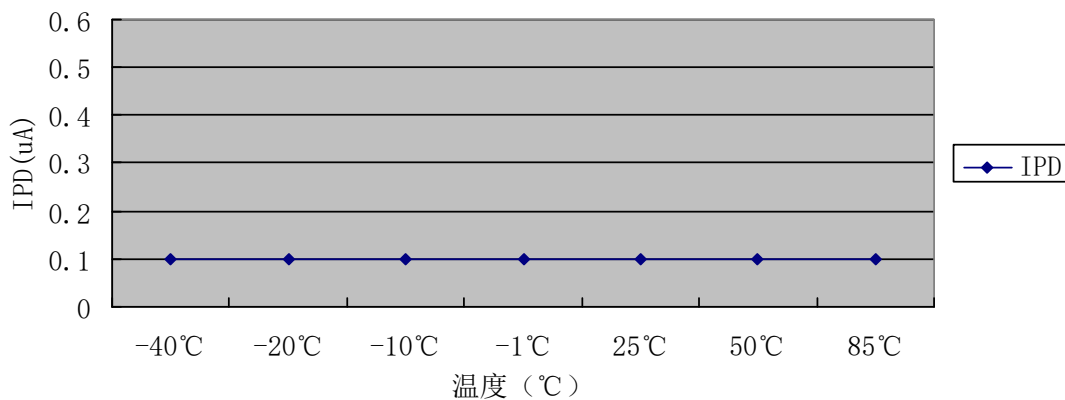
休眠电流与温度曲线
