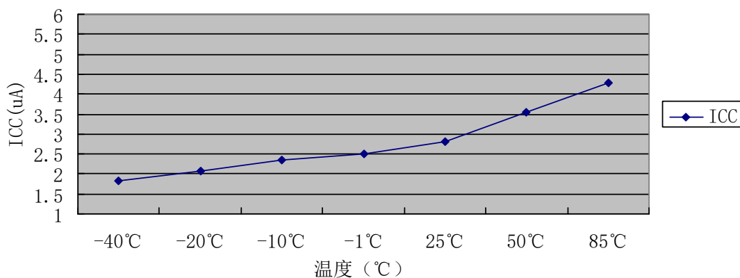
动态功耗与温度曲线
