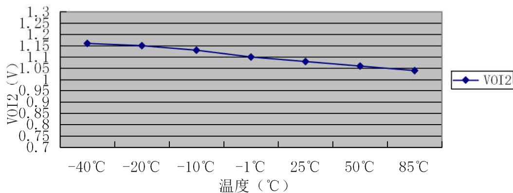
短路保护电压与温度曲线
