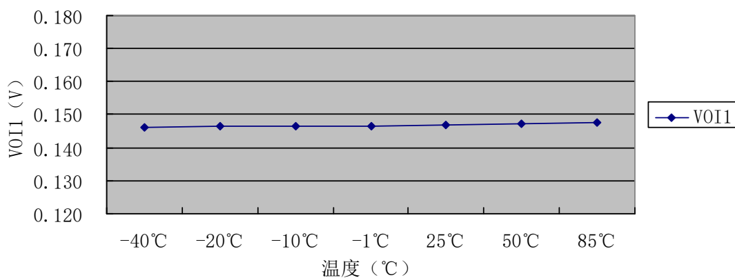
过流保护电压与温度曲线
