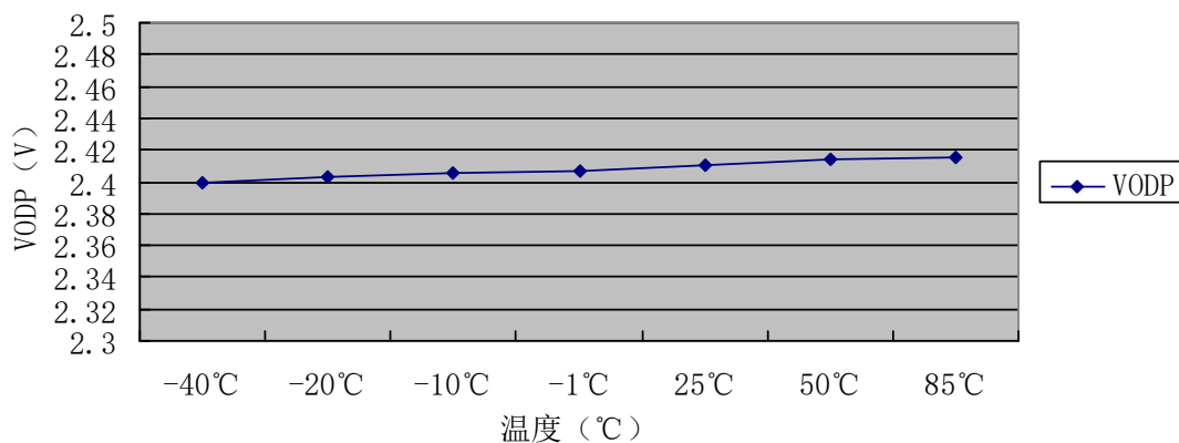
过放电压与温度曲线
