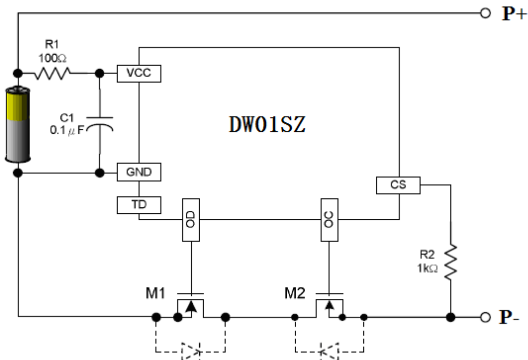
单节锂离子电池保护电路图
